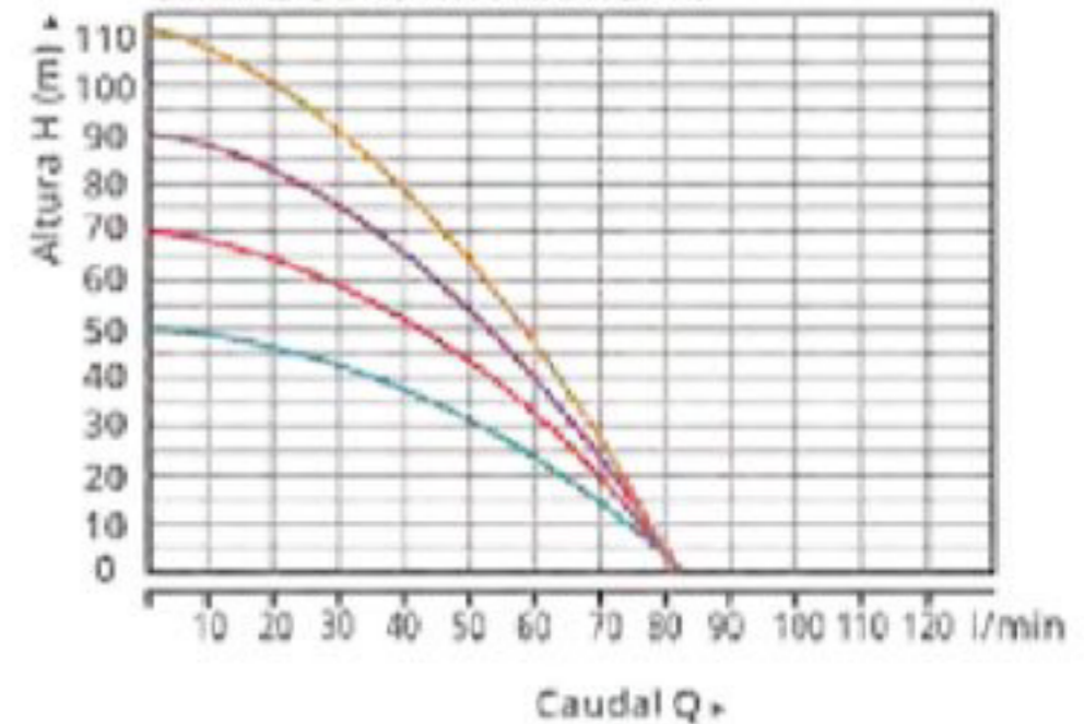
CURVAS DE FUNCIONAMIENTO
