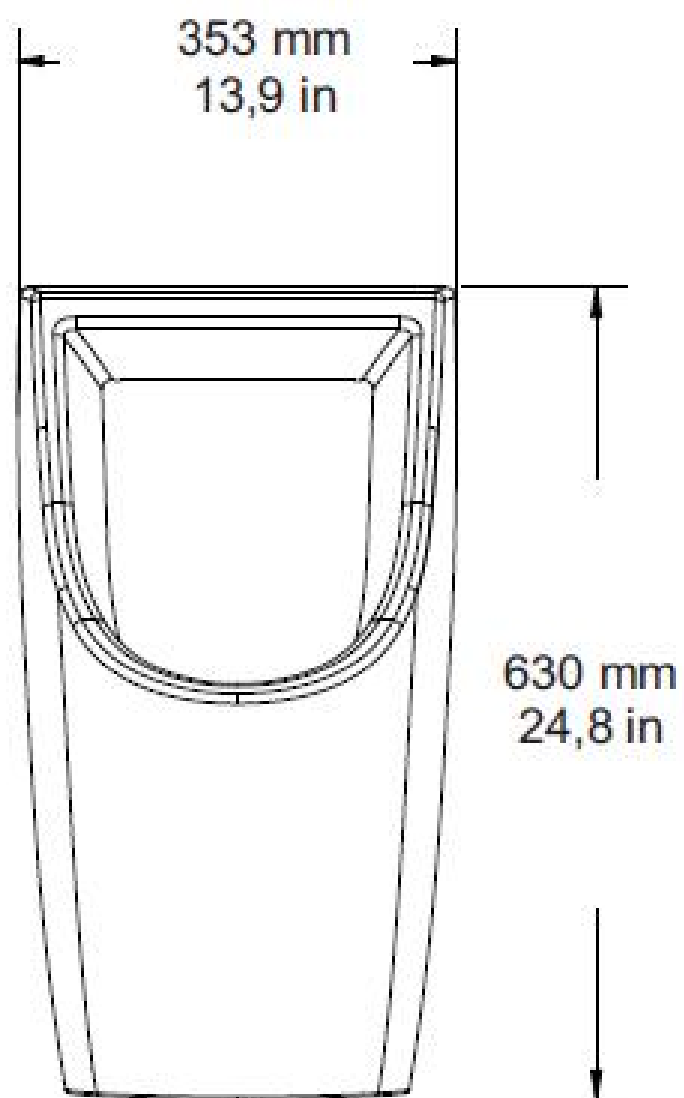
Medidas Referenciales / Estimated Dimensions, Acot. mm [pulg.] / Dim. mm [inch.]
